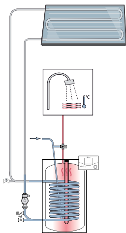
Sistema solar sem vaso de expansão
