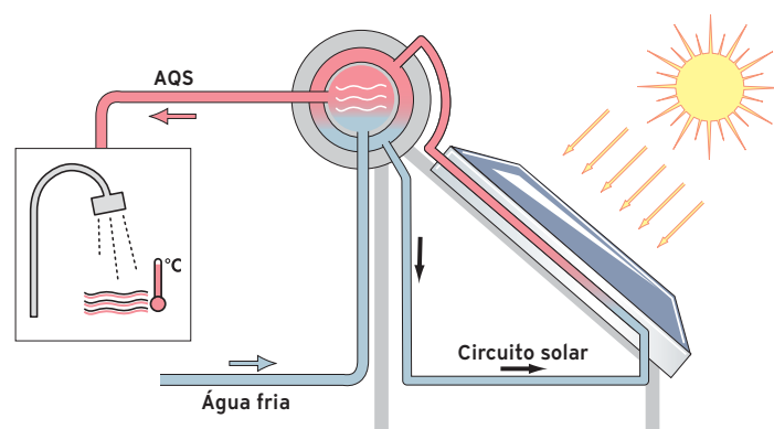
Esquema de funcionamento do auroSTEP pro
