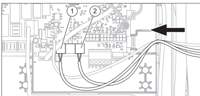
1 Διάυλος eBUS 2 24 V-S20
